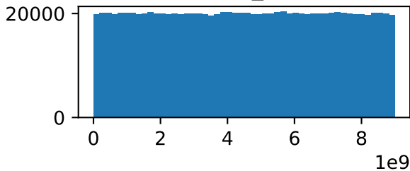
comoving_volume
