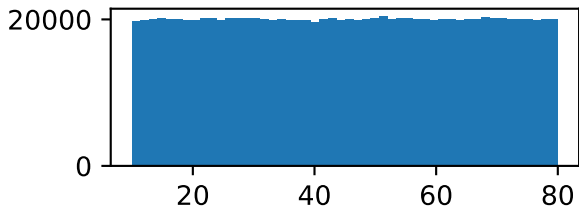
srcmass1
