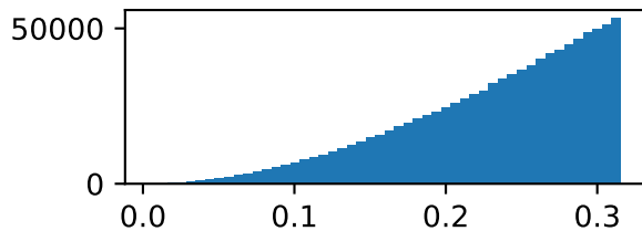
redshift
