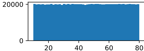
srcmass2
